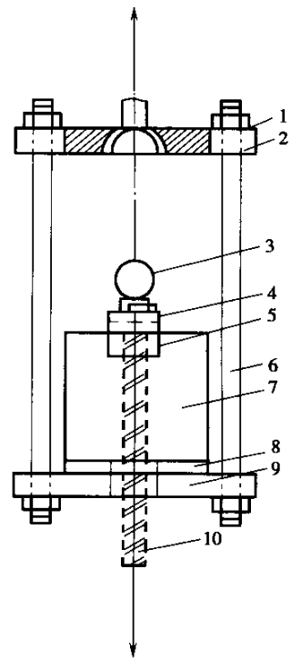
图 C.0.2-2 握裹力试验装置示意
