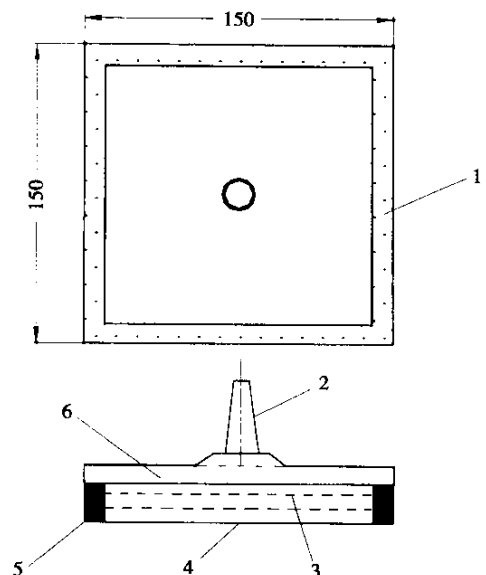
图 E.1.2-2 真空吸盘(尺寸单位:mm) 1-橡胶封圈;2-吸水嘴;3-骨架层;4-过滤层;5-封圈;6-密封层
