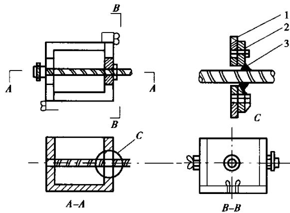
图 C.0.2-1 握裹力试验用试模
