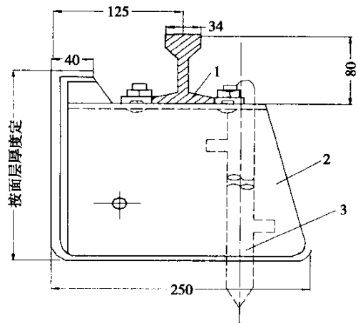
图 7.2.2 轨道模板(尺寸单位:mm)
