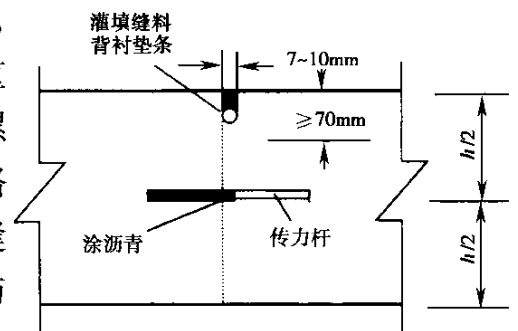
图 9.1.2 横向施工缝构造示意图
