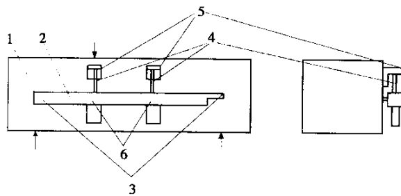
图 D.1.3-2 挠度测量装置示意图
