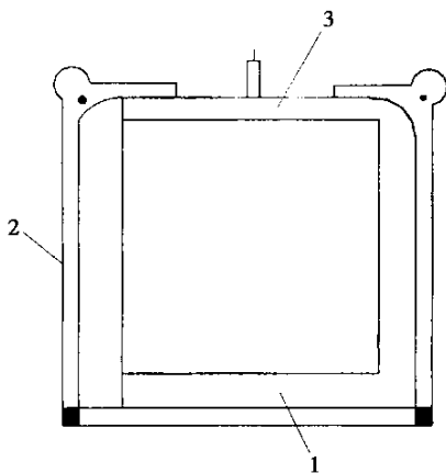
图 E.1.2-1 真空吸盘固定架 1-试模;2-吸盘固定架;3-吸盘
