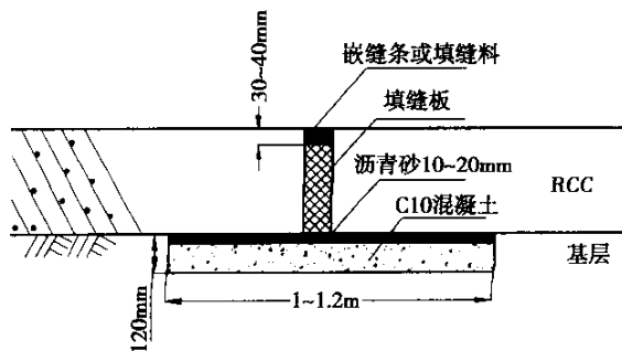
图 7.6.8-1 混凝土枕垫式胀缝
