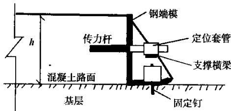
图 7.2.1-2 工作缝端模侧立面
