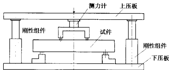
图 D.1.3-1 刚性组件装置
