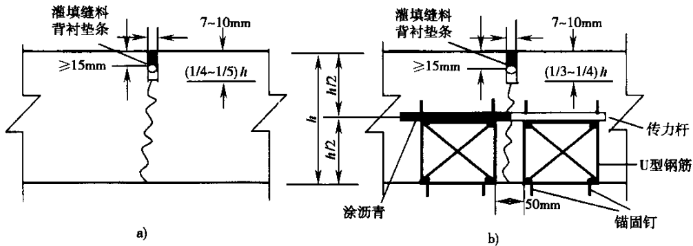
图 9.1.3 横向缩缝构造 a)假缝型;b)假缝加传力杆型
