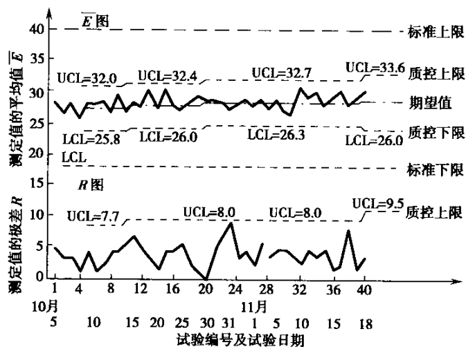
图 A.2.3-1 工程质量指标管理图示例(抗压强度, MPa) (图中每一个点为每次测定的三个试件的平均值 \bar{E} 或极差 R )
