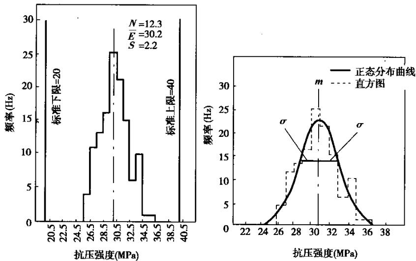
图 A.2.3-2 工程质量检测结果的直方图及正态分布曲线示例
