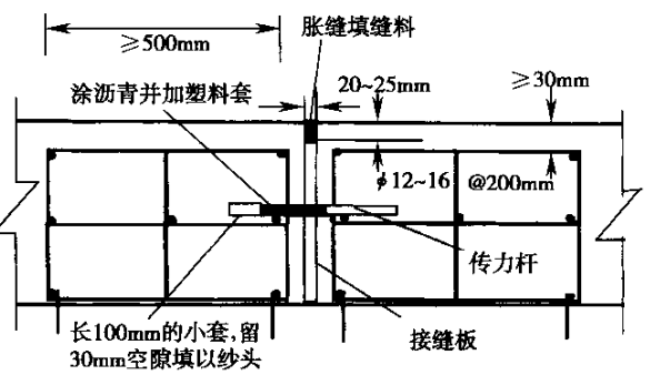
图 9.1.4 胀缝构造示意图
