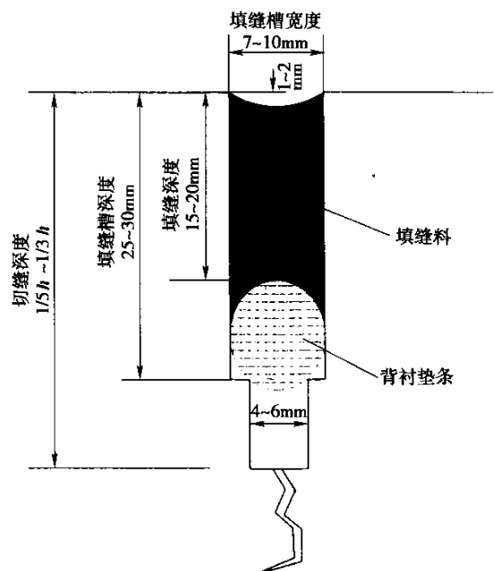
图 9.1.6 缩缝切缝、填缝(槽)、垫条细部尺寸
