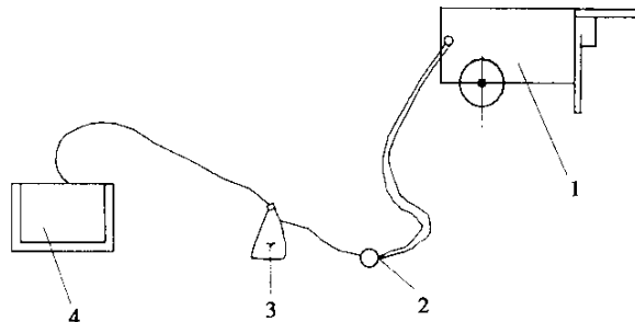
图 E.1-3 混凝土真空脱水系统连接图
