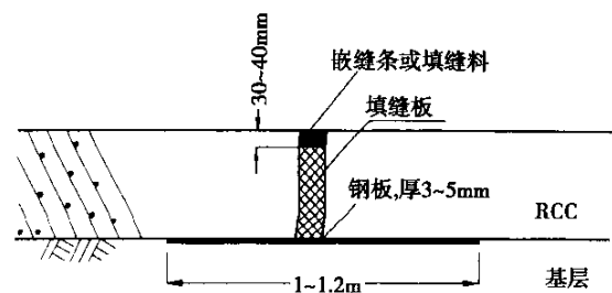
图 7.6.8-2 钢板枕垫式胀缝
