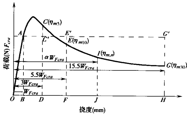
图 D.1.5 荷载—挠度曲线及弯曲韧度指数
